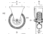
寸法図
