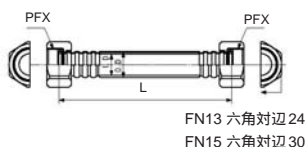
ロングフレキ10M巻(ステンレスフレキチューブ) 肉厚0.3mm
