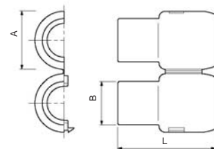
袋ナットカバー
